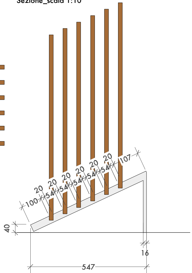
Sezione_scala 1:10
