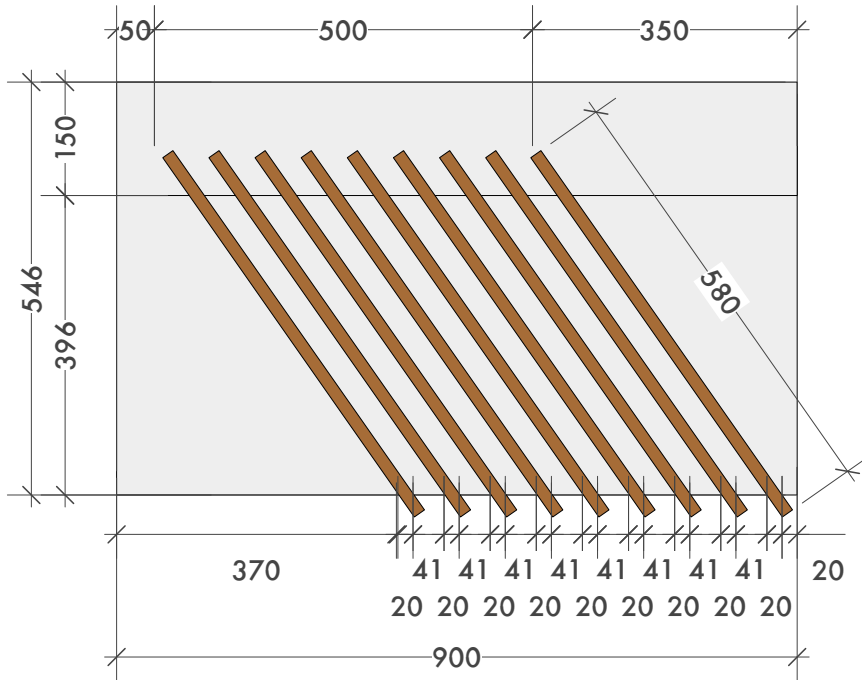
Pianta_scala 1:10
