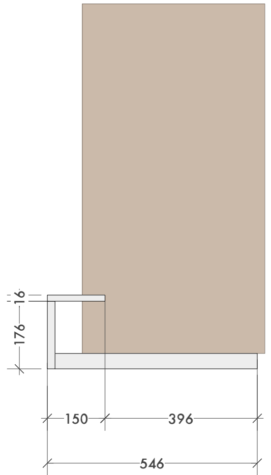
Sezione_scala 1:10
